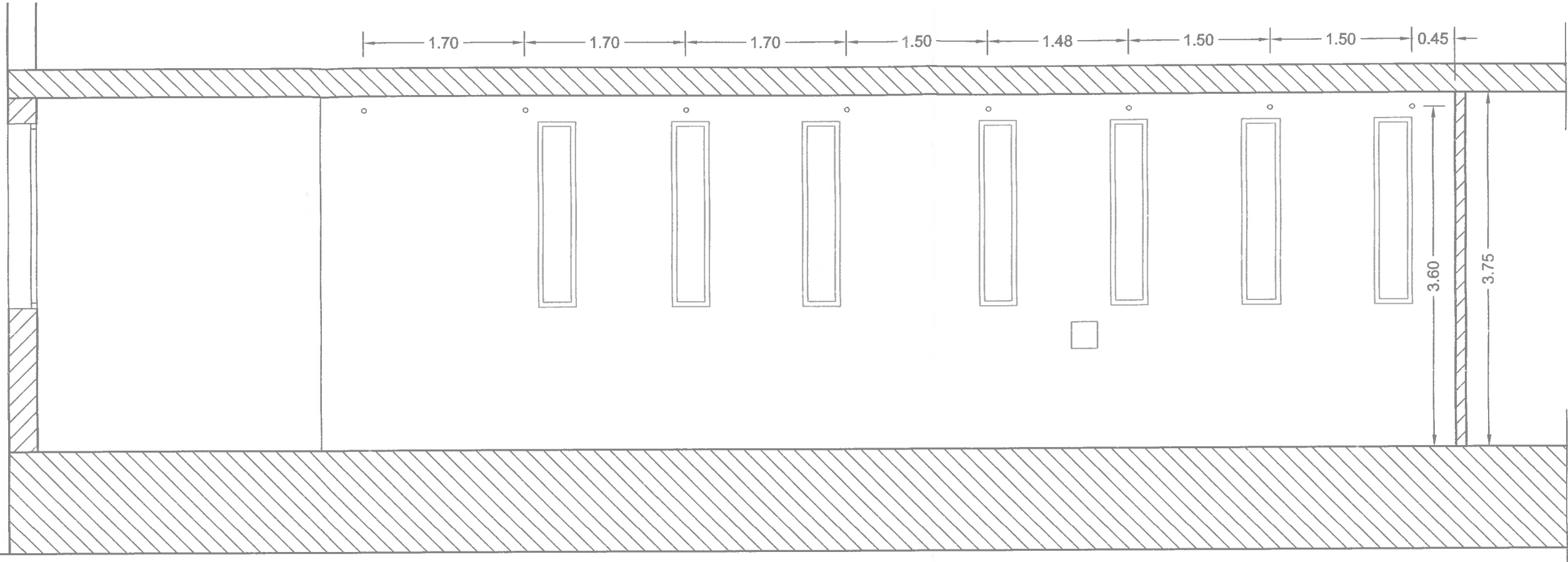
ALZADO "A"
